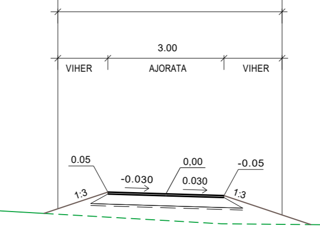
TYYPPIPOIKKILEIKKAUS KLV PENKEREELLÄ 1:100
