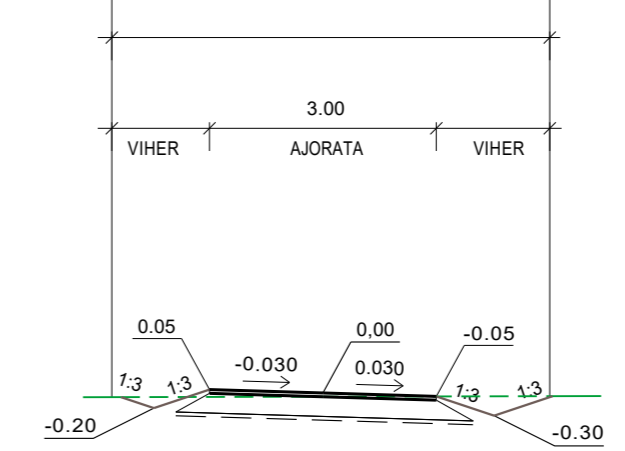
TYYPPIPOIKKILEIKKAUS KLV LEIKKAUKSESSA 1:100
